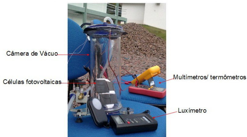
Figura 1 – Fotografia dos componentes do sistema utilizado.
