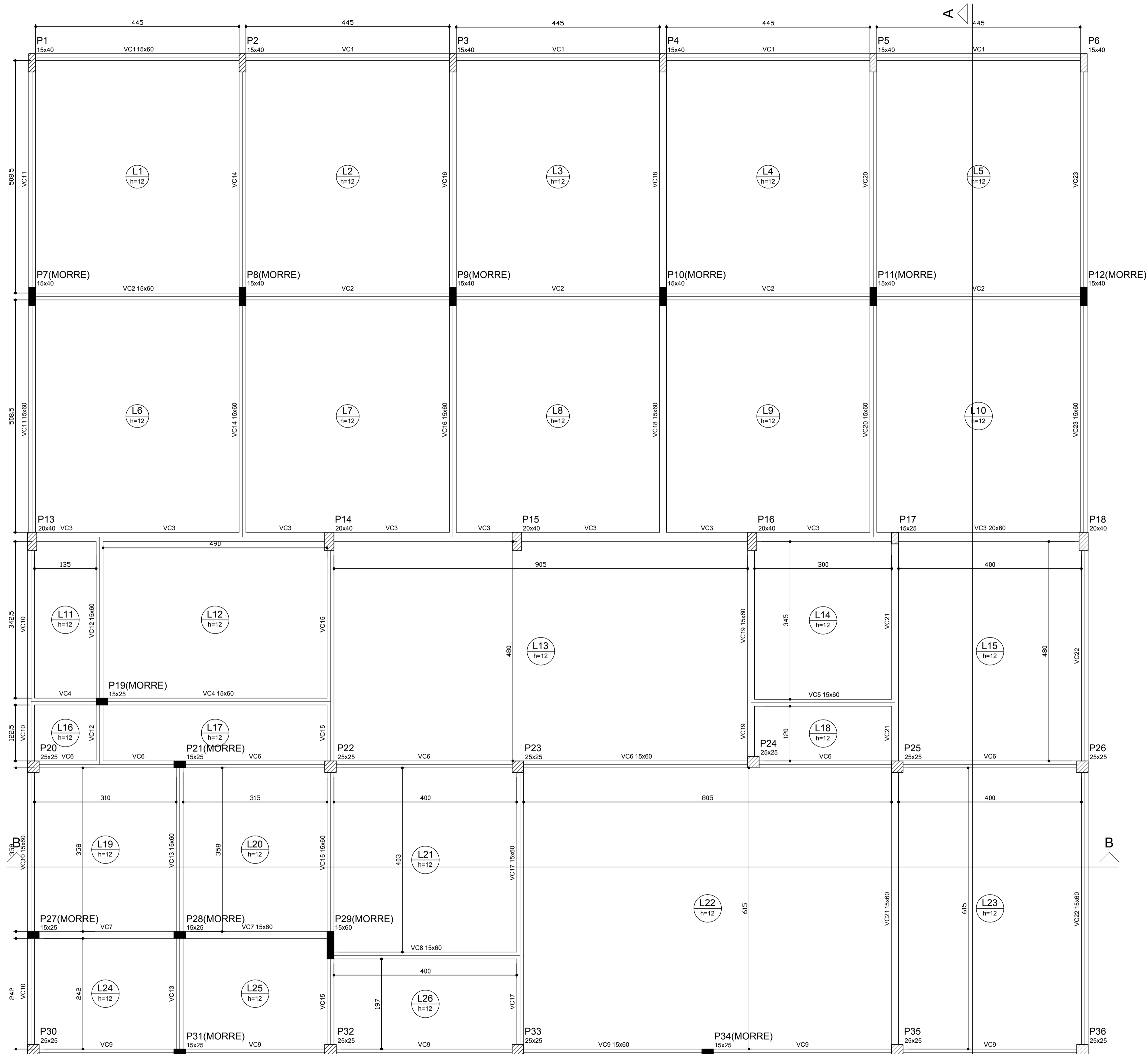
Forma do pavimento Térreo escala 1:50
