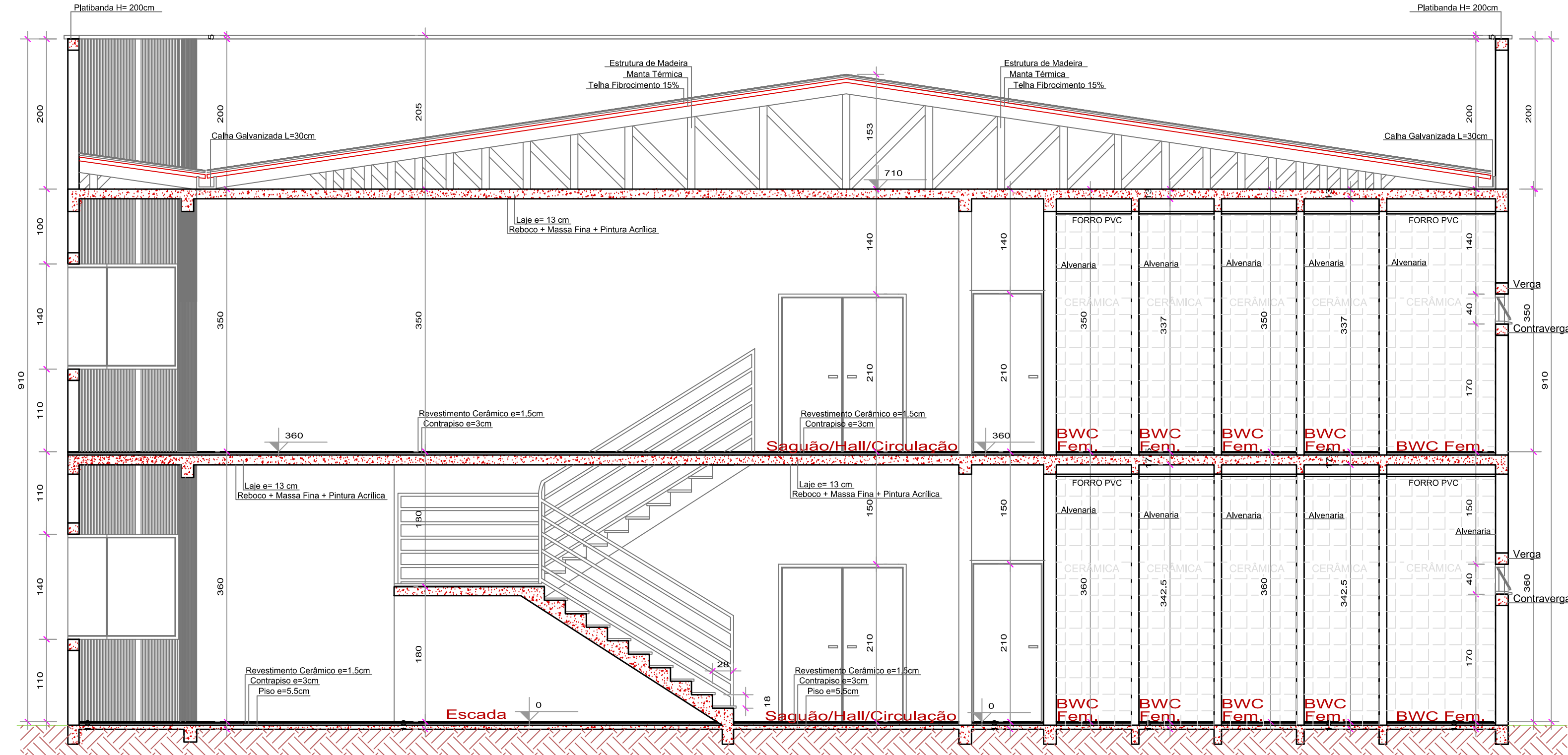
CORTE BB
