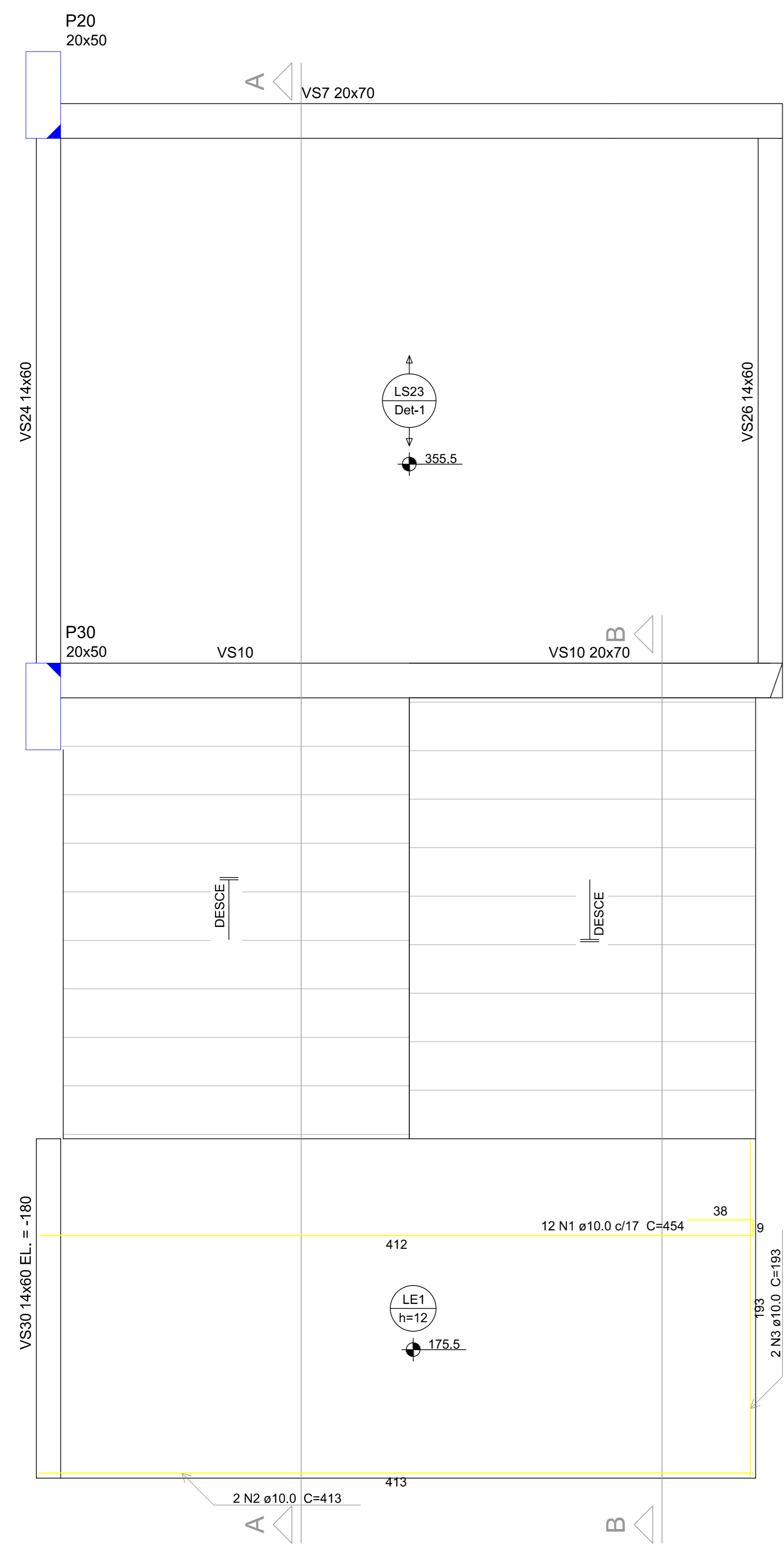
Armação positiva da escada E1 escala 1:25
